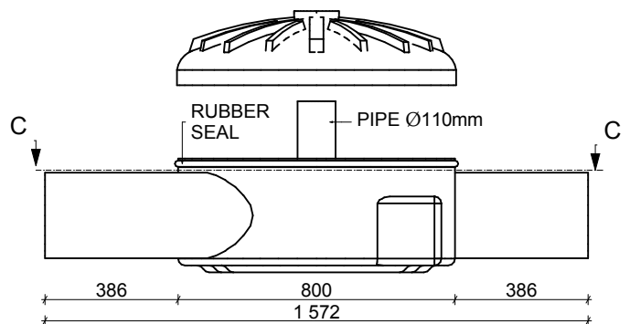
ELEVATION B
